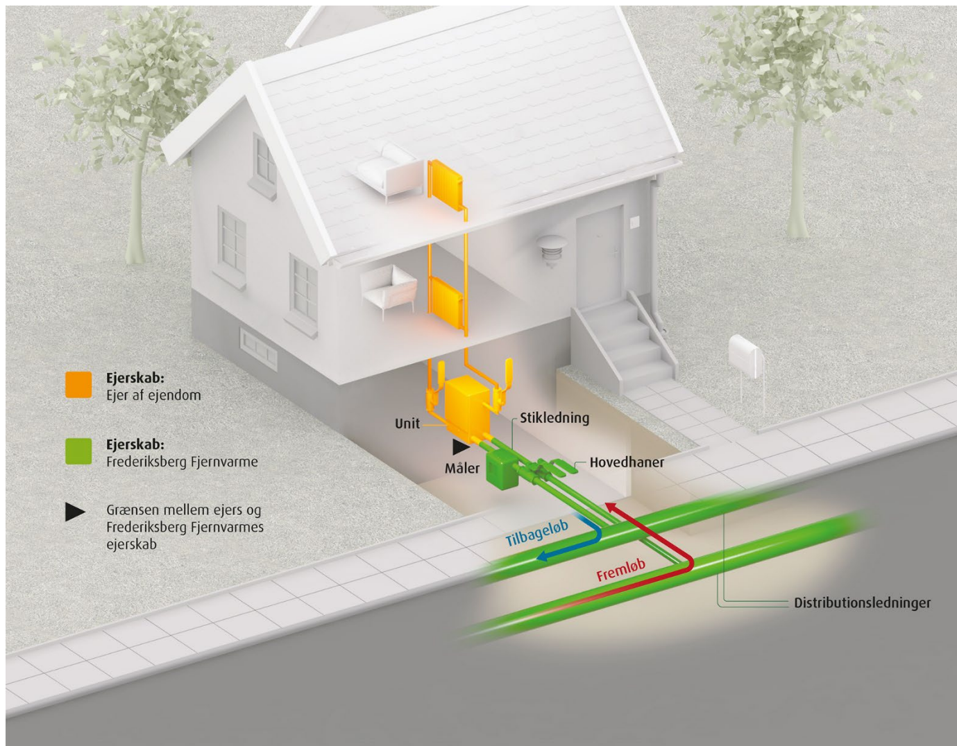
Illustration 1: Fjernvarmeinstallationer
