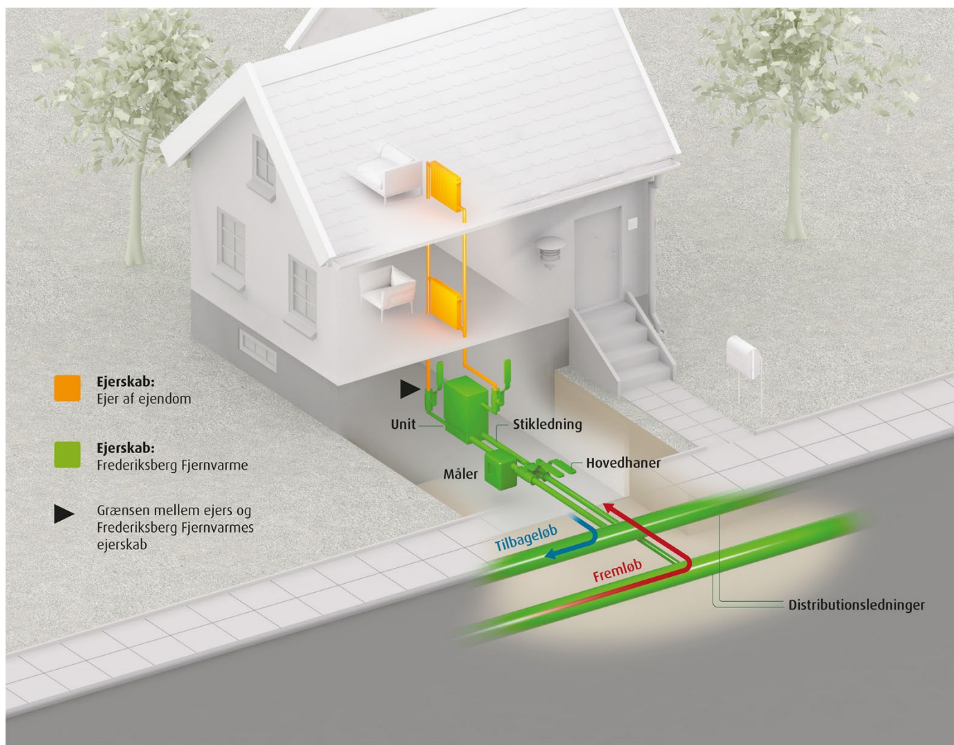
Illustration 2: Fjernvarmeinstallation med tilvalg af Unit
